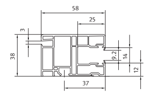
Maxi Führungsschiene K51/K52/RS52 einfach | Artikel 3006011
