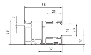
Maxi Führungsschiene K51/K52/RS52 einfach | Artikel 3006011
